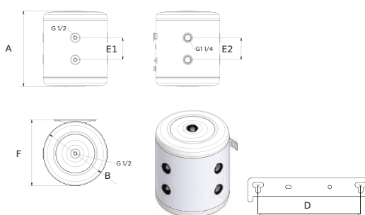
BF100 - Dimensões
