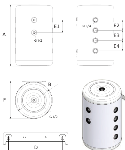
BF080 - Dimensões
