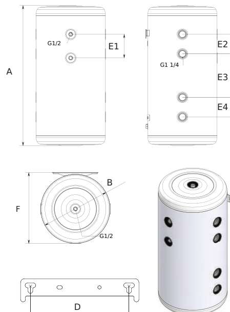
BF100 - Dimensões
